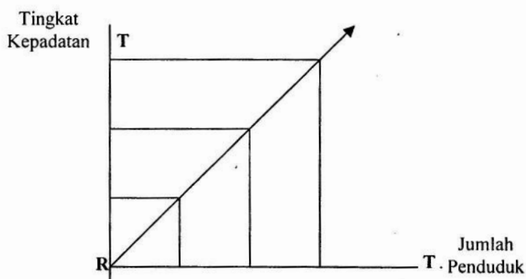
Gambar 5.11. Contoh Grafik Hubungan Positif
