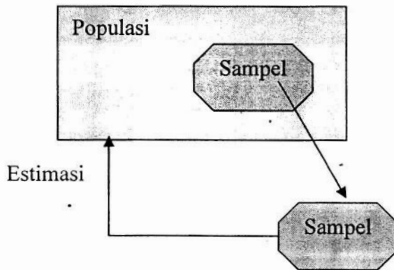
Gambar 6.1. Hubungan Populasi dan Sampel
