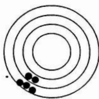
Reliabilitas tinggi dan validitas rendah
