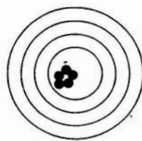
Reliabilitas tinggi dan validitas tinggi
