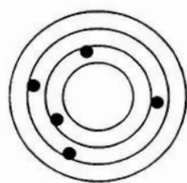
Reliabilitas rendah dan validitas rendah
